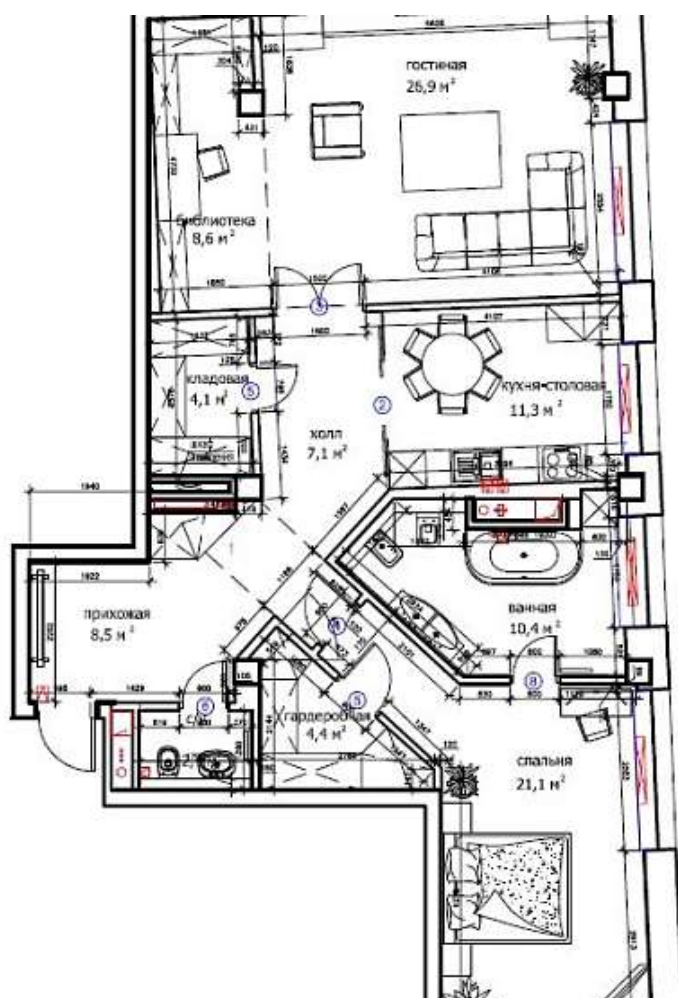
Планировка согласно дизайн-проекту М 1:75
