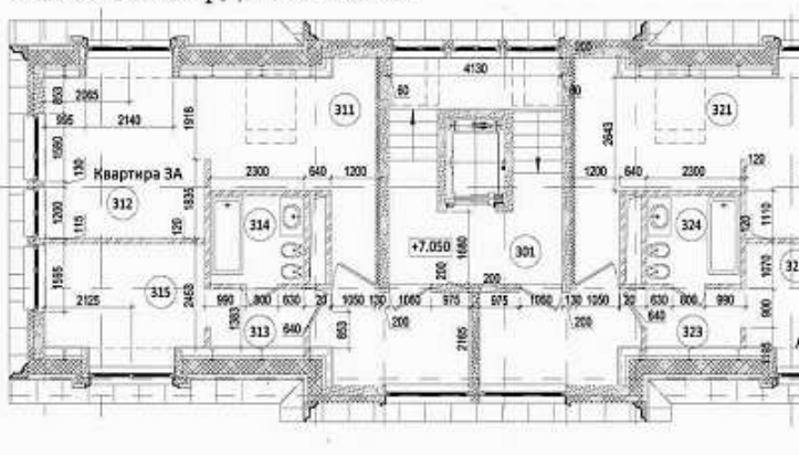
План мансардного этажа
