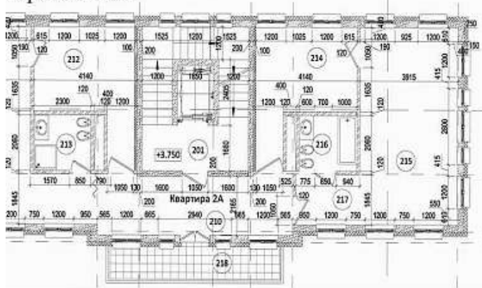
План второго этажа
