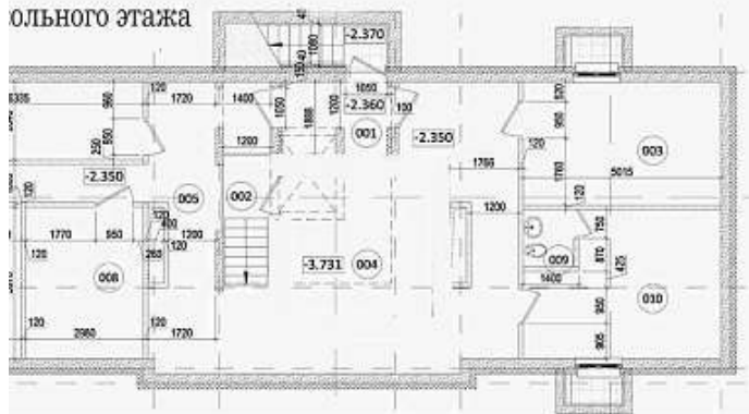
План первого этажа
